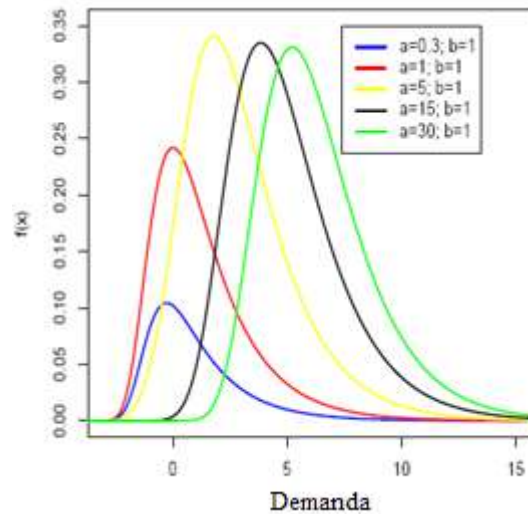
Figura 4. Distribución Moyal
